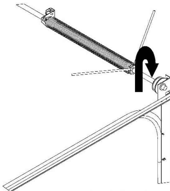
Fig.20. Tensado de muelles.
