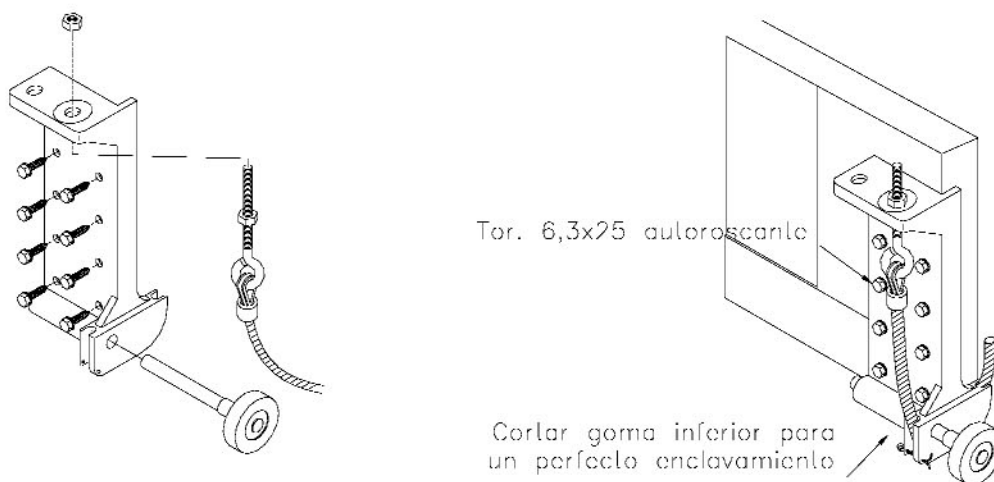
Fig. 9. Montaje placa base.
