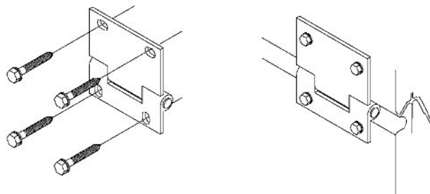
Fig.10 Instalación de portarrodillos laterales y bisagras intermedias.
