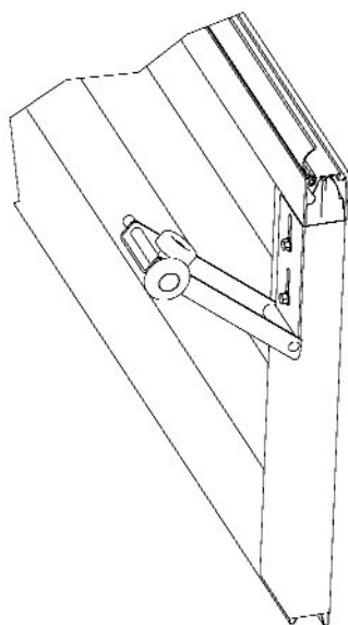
Fig.12. Portarrodillo superior D150
