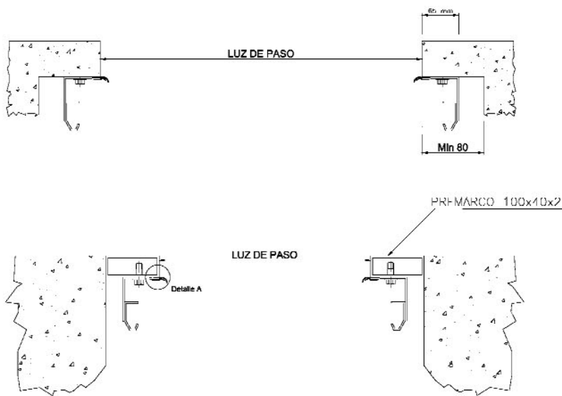
Fig.2 Disposición del premarco
