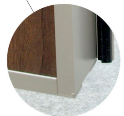
Hoja de 45 mm. Chapa de aluminio de 1.5 mm. - 2.0 mm.
