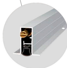
Cortavientos inferior automático
